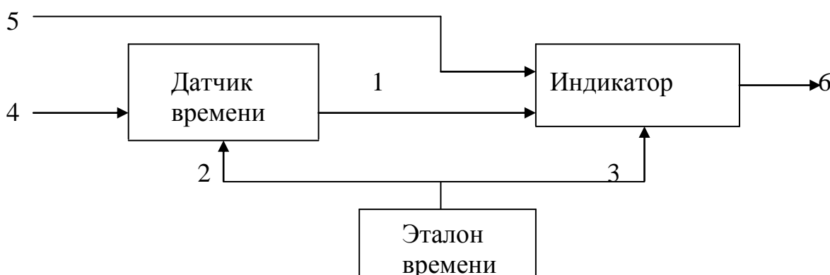
Рисунок 2 – Структурная схема системы «синхронизируемые часы»
